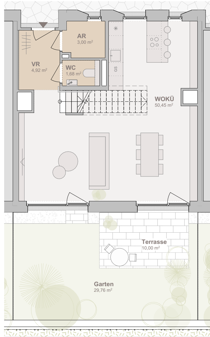
Erdgeschoss
